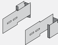
STUD CLIPS
